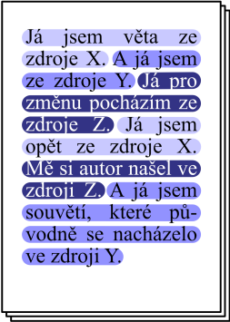
Obrázek 1: Mozaikové plagiátorství
